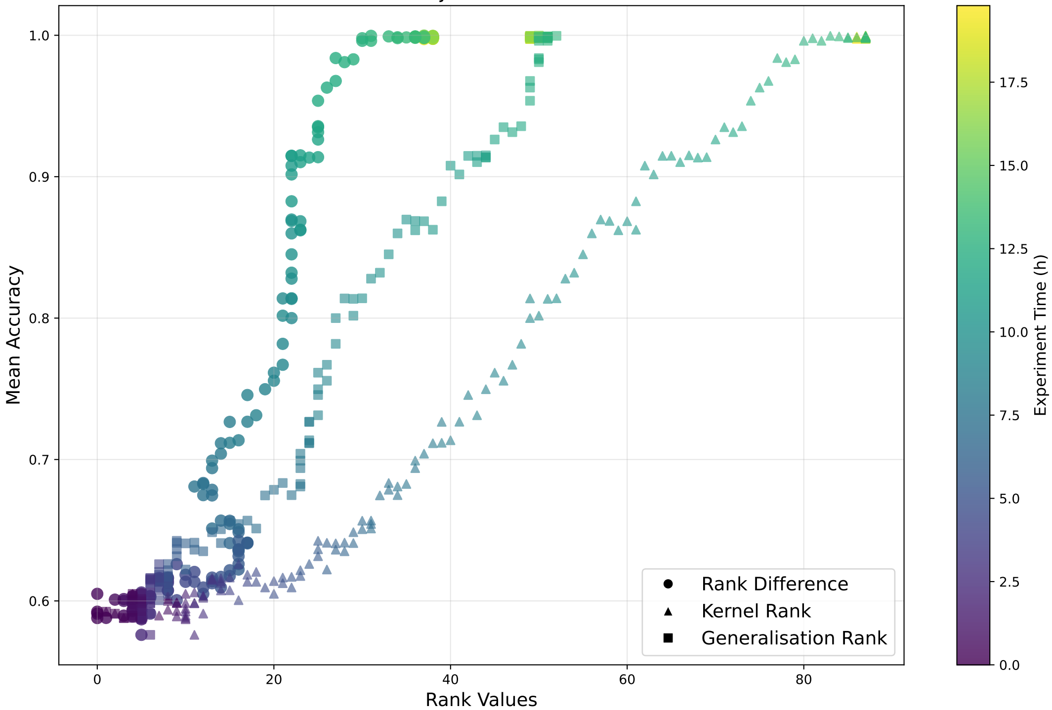
Rank Trajectories - E. coli
