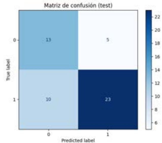
Figura 8: Matriz de confusión en el conjunto de prueba para el Random Forest de color.
