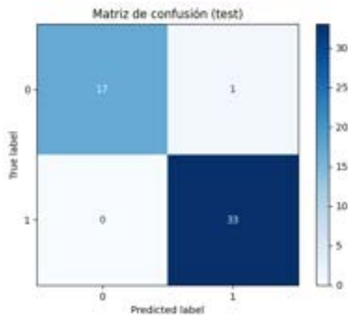
Figura 21: Matriz de confusión del ensamblado en test.
