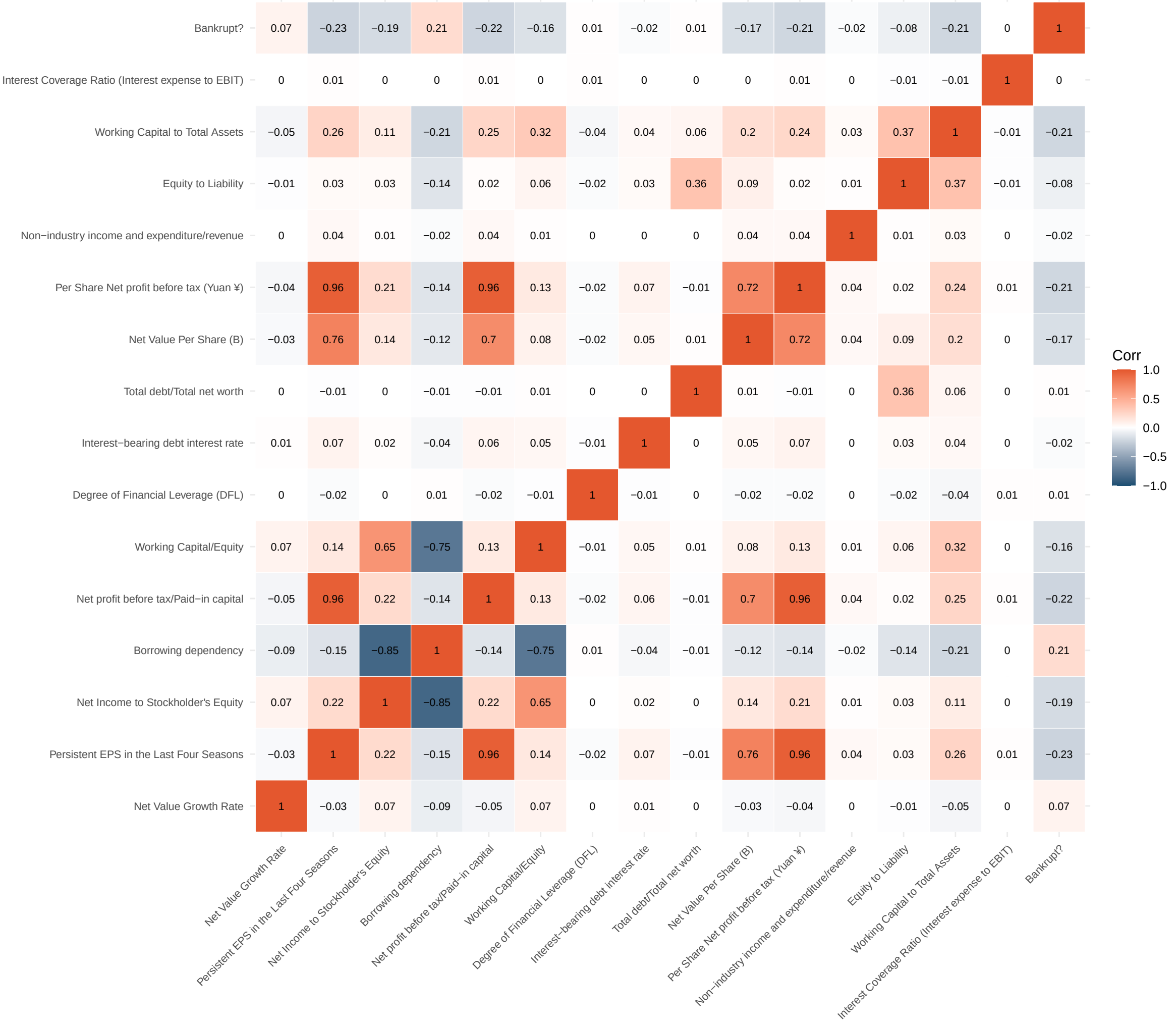
Matriz de correlación — Top 15 variables (train)
