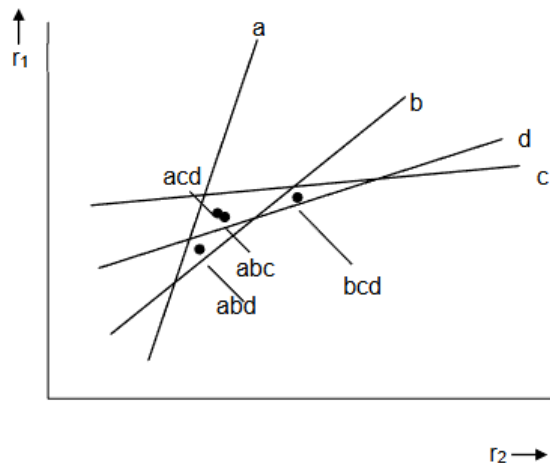
Abb. 5: Graphische Copolysmerisationsparameterbestimmung.[polyskript]
