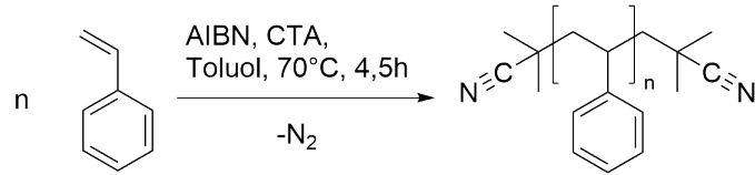
Abb. 4: Reaktionsgleichung zur Synthese von Polystyrol über RAFT.
