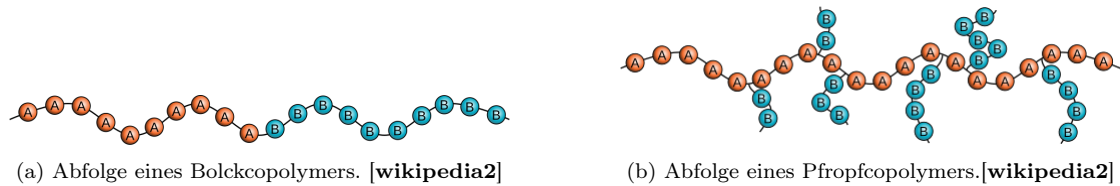
Abb. 11: Abfolgen eines Block- sowie Pfropfcopolymers.
