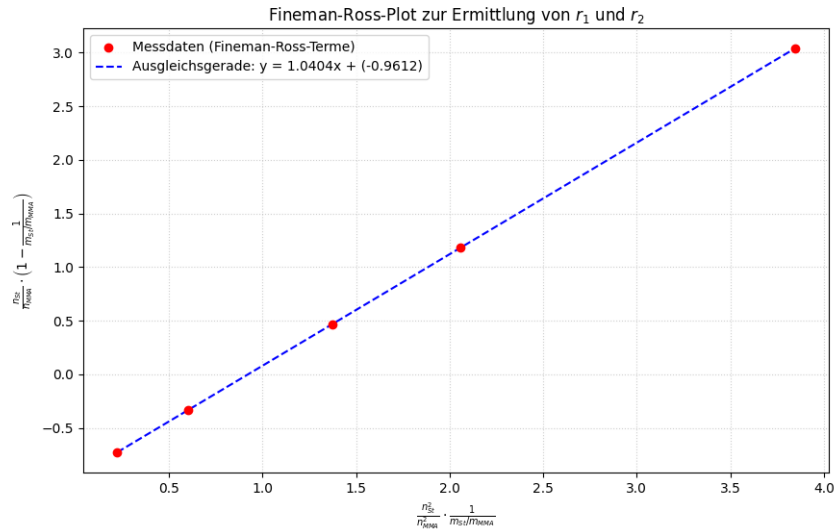
Abb. 9: Der Graph zeigt die Graphische bestimmung der Copolymerisationskonstanten über die Fineman Methode.
