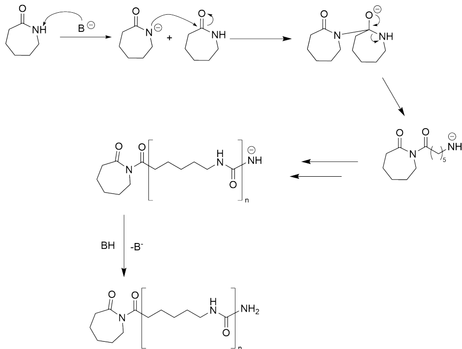
Abb. 6: Die Abbildung zeigt die ringöffnende Polymerisation von Caprolactam zu Nylon-6.
