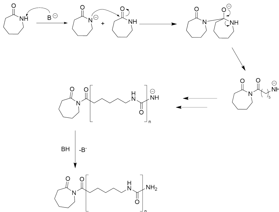
Abb. 7: Die Abbildung zeigt die ringöffnende Polymerisation von Caprolactam zu Nylon-6.
