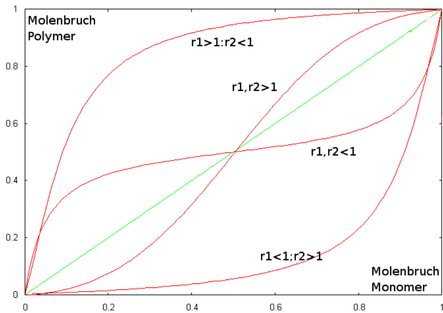
Abb. 13: Verläufe der Copolymerisationskurve für unterschiedliche r -Werte. [2]
