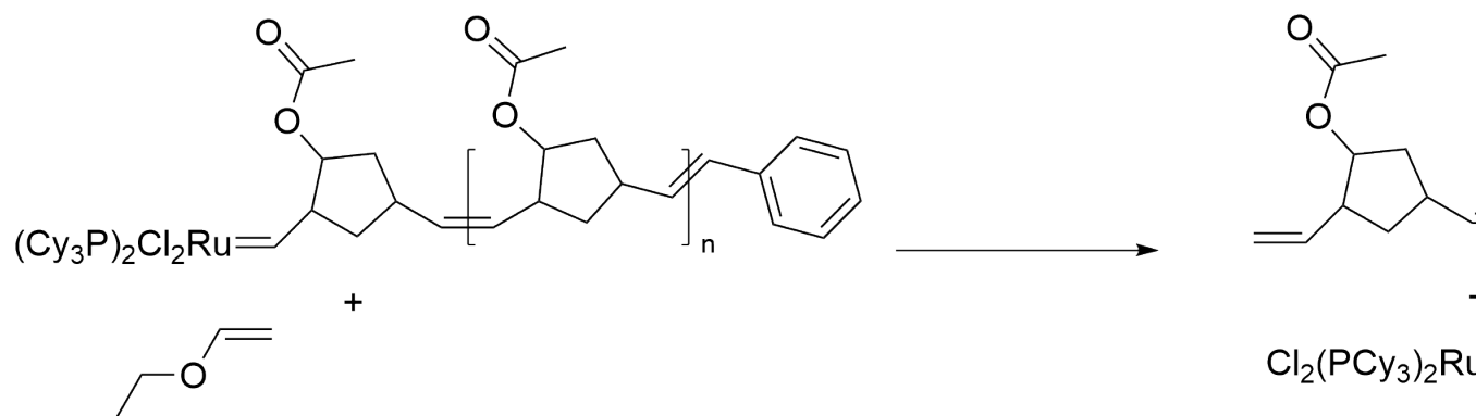
Abb. 9: Reaktionsgleichung des Abbruchreaktion zwischen dem Grubbs-Polymer und Ethylvinylether.
