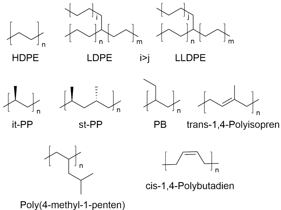
Abb. 8: Abgebildet sind die Strukturen der Polymere.
