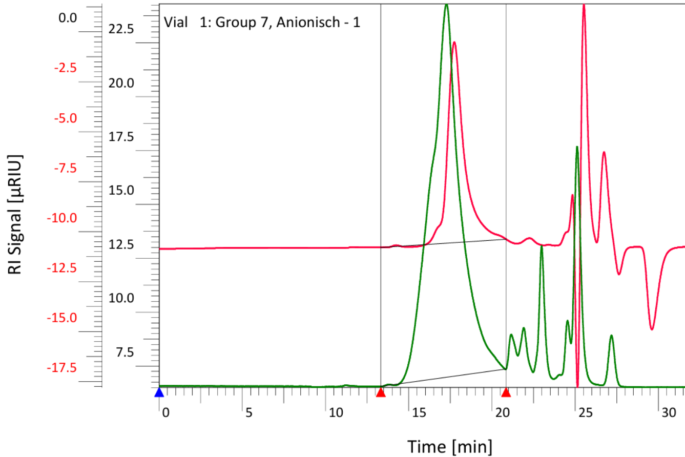
Abb. 4: Auftragung des RI-Signals auf die Zeit für die anionische Copolymerisationsprobe.
