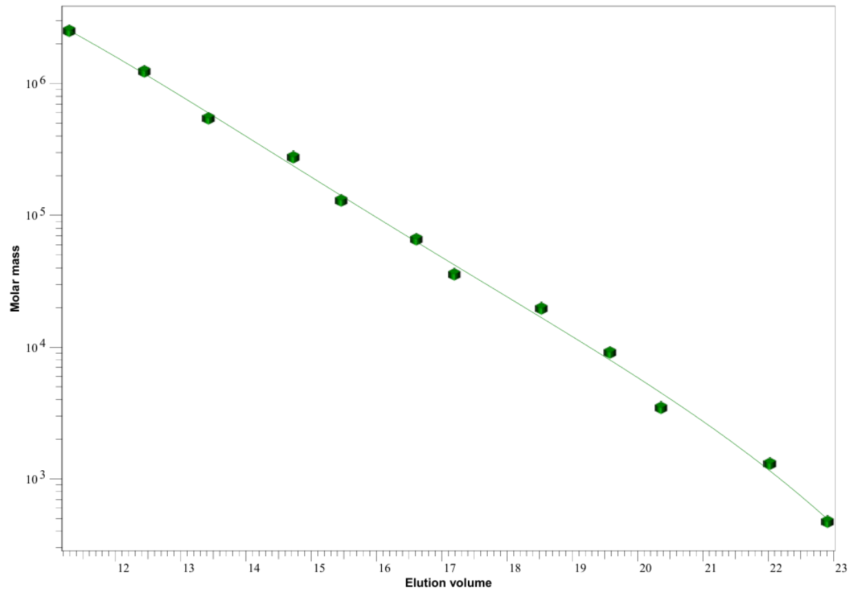
Abb. 2: Logarithmische Auftragung der unterschiedlichen Molekulargewichte der Polystyrolstandards auf das Elutionsvolumen.
