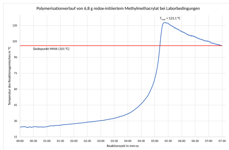
Abb. 3: Die Abbildung zeigt den Norrish-Trompsdorff-Effekt Graphisch dargestellt.[ wikipedia ]
