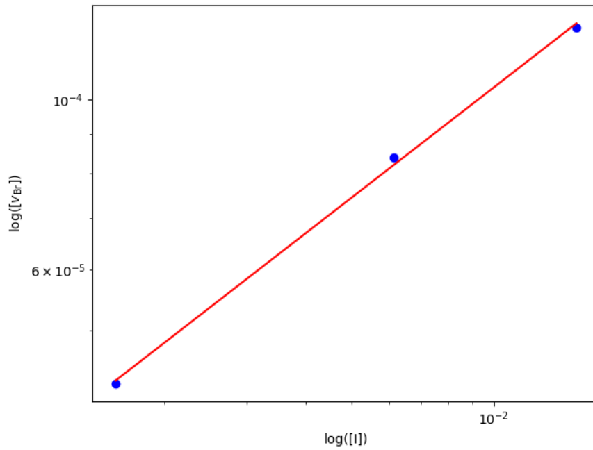
Abb. 7: Doppellogarithmische Auftragung der Bruttogeschwindigkeit v_{Br} auf die Initiatorkonzentration [I] .
