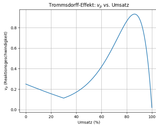
Abb. 11: Visualisierung des Norish-Trommsdorff-Effekts.
