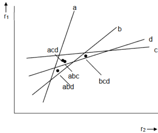
Abb. 6: Graphische Copolymerisationsparameterbestimmung. [1]
