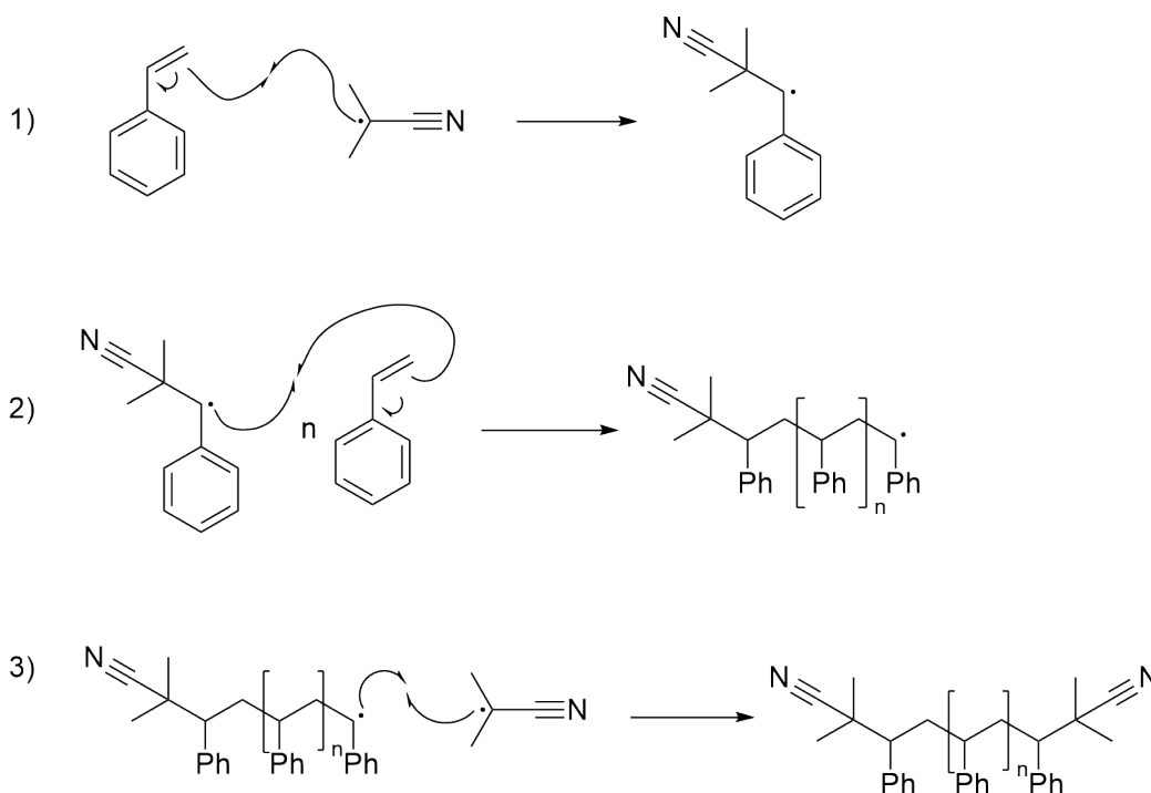
Abb. 2: Die Abbildung zeigt die radikalische Polymerisation mit Start, Wachstum und Abbruch. Als Abbruch wurde hier eine Rekombination als Beispiel gewählt.
