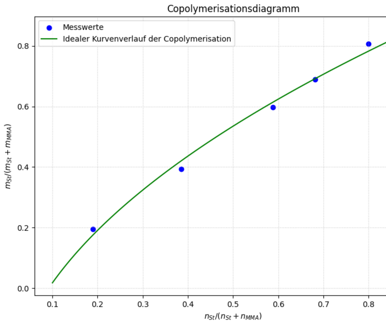
Abb. 10: Die Abbildung zeigt das Copolymerisationsdiagramm der Copolymerisation von Styrol und MMA
