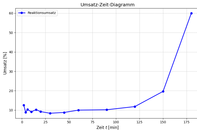
Abb. 2: Die Abbildung zeigt den Umsatz in % aufgetragen auf die Reaktionsdauer.
