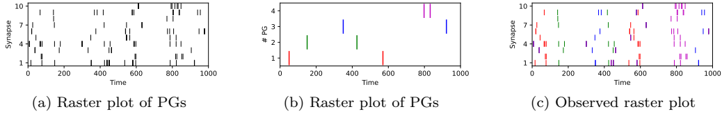
FIGURE 5 : Un exemple de “raster plot” synthétique est généré dans (a) comme la combinaison de PGs dont le timing et l’identité sont déterminés dans (b), ici une superposition de 4 PGs projetés sur l’espace synaptique de 10 neurones et à une fréquence moyenne de 3 Hz pendant 1000 ms. En observant les spikes de (a), le modèle décode l’identité et le timing des PGs dans (b), ce qui nous permet de colorer les spikes dans (c).
