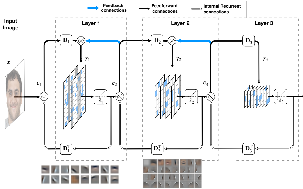
FIGURE 2 : Dans [Bou+21], nous proposons un modèle de traitement hiérarchique de l'information visuelle (ici de 3 couches). De façon similaire à des réseaux de neurones convolutionnels classiques, chaque couche est constituée de canaux auxquels sont attribués des champs récepteurs. Toutefois, contrairement aux réseaux classiques, l'apprentissage est ici bio-mimétique, c'est-à-dire qu'au lieu d'opérer une retro-propagation (globale) du gradient, les opérations sont toutes locales et s'opèrent de proche en proche. Cet apprentissage non-supervisé est possible par l'introduction d'une contrainte de régularisation assurant la parcimonie de la représentation. On observe l'émergence de champs récepteurs sensibles à des bords orientés dans la première couche, de façon similaire à ce qui est observé dans le cortex visuel primaire. De façon plus surprenante, quand on apprend le réseau sur une base d'images de visages, on observe l'émergence de cellules sensible à des composantes indépendantes : bouche, yeux, contours allongés, ... (Reproduit de [BoutinFranciosiniChavaneRuffierPerrinet19] selon les termes de la Creative Commons Attribution License, © The Authors 2017.)
