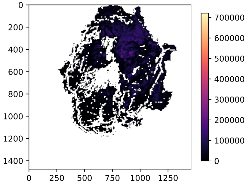
ember flux
