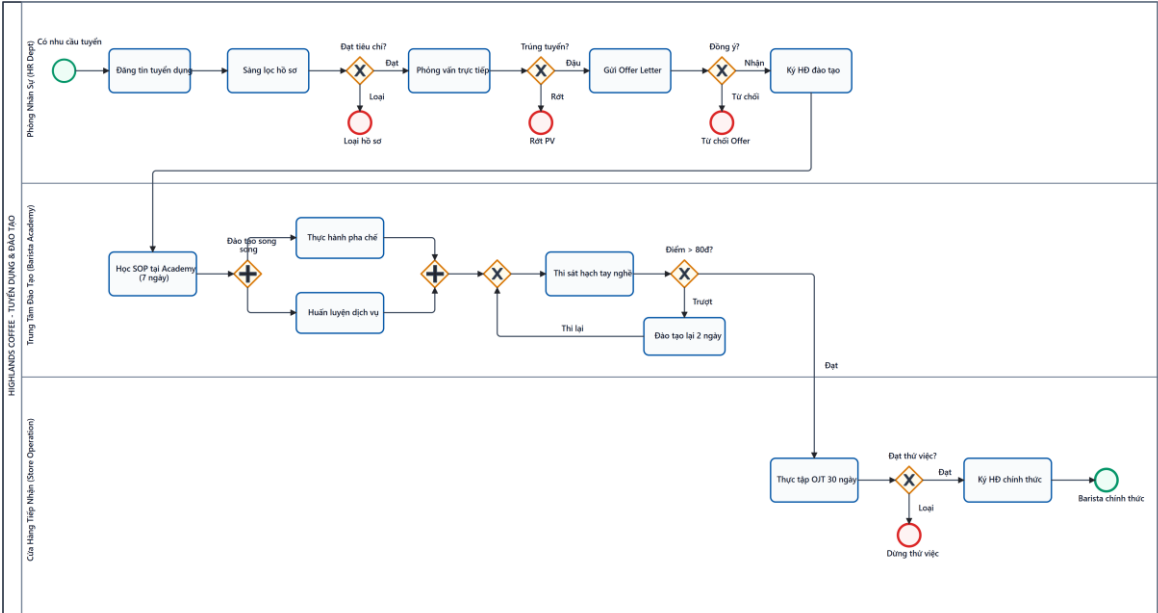
Hình 2.15: Sơ đồ BPMN 2.0 Quy trình Tuyển dụng & Đào tạo Barista Mới (P09)
