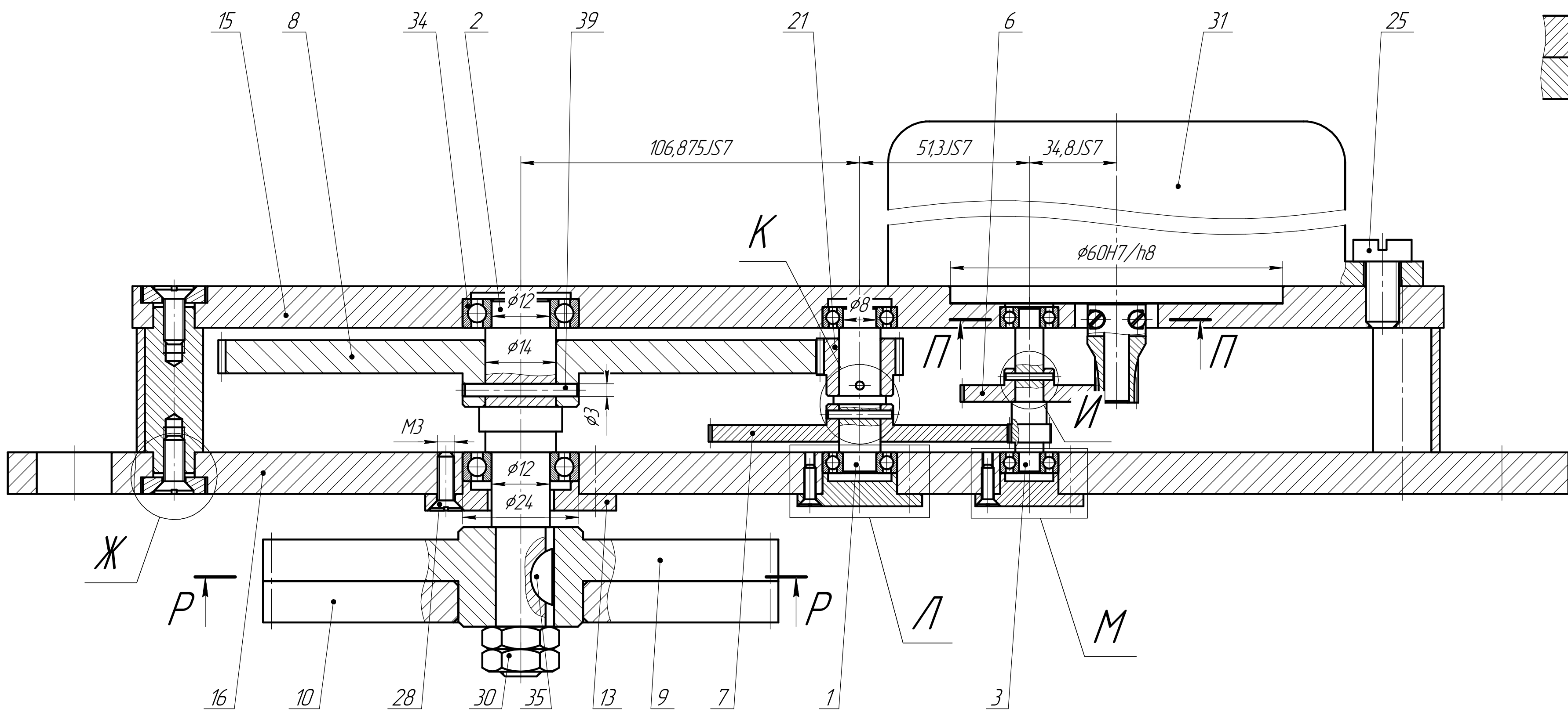
A-A (2:1)
