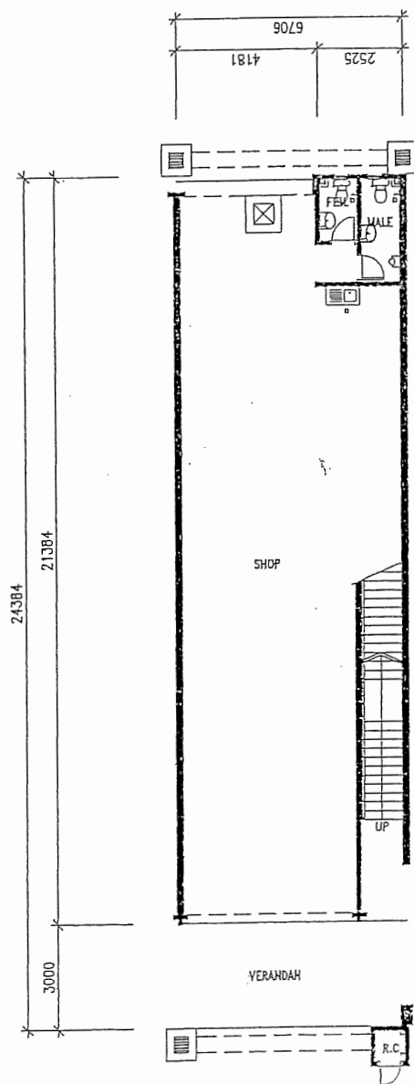
PELAN TINGKAT BAWAH
