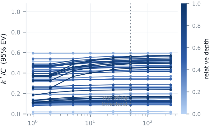
timm_resnet50.gluon_in1k
