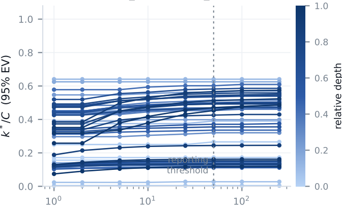
timm_resnet50.tv2_in1k
