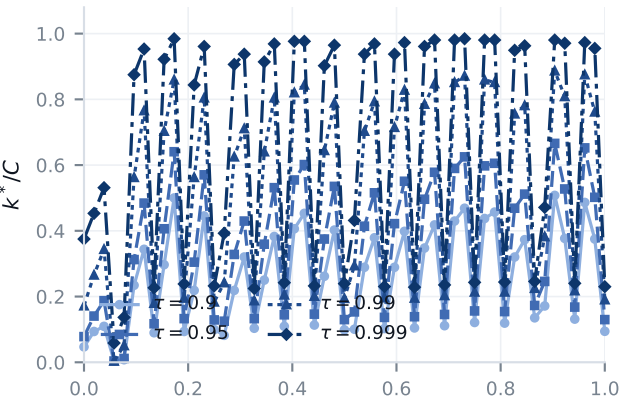
timm_resnet50.a1_in1k
