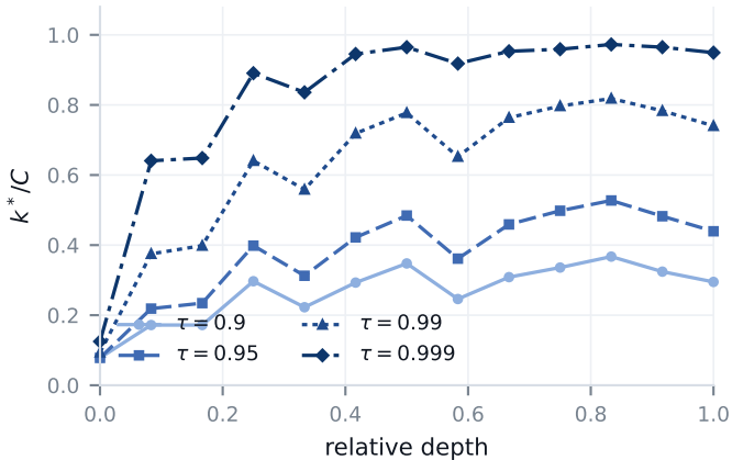
vgg16_bn
