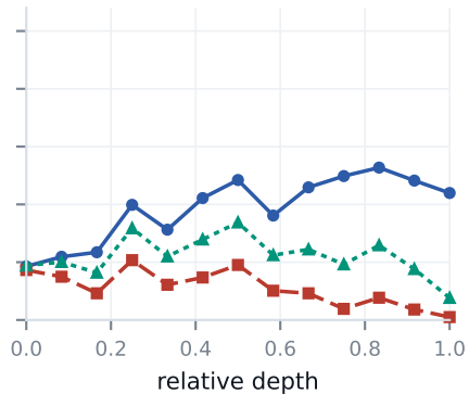
VGG-16 (BN)
