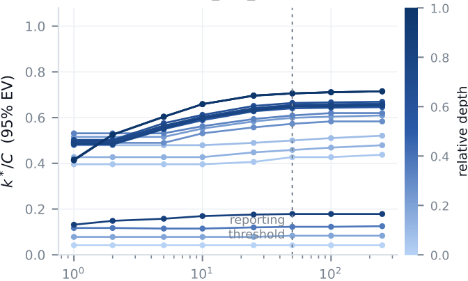
convnext_tiny_random
