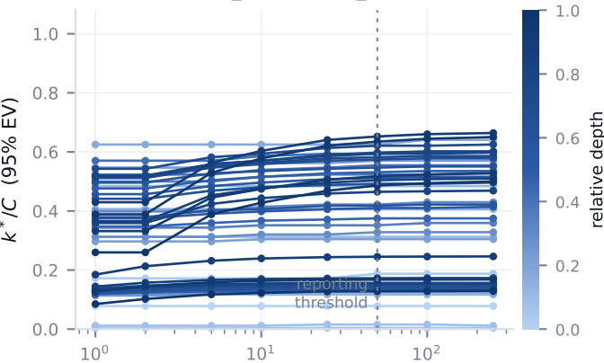
timm_resnet50.a1_in1k
