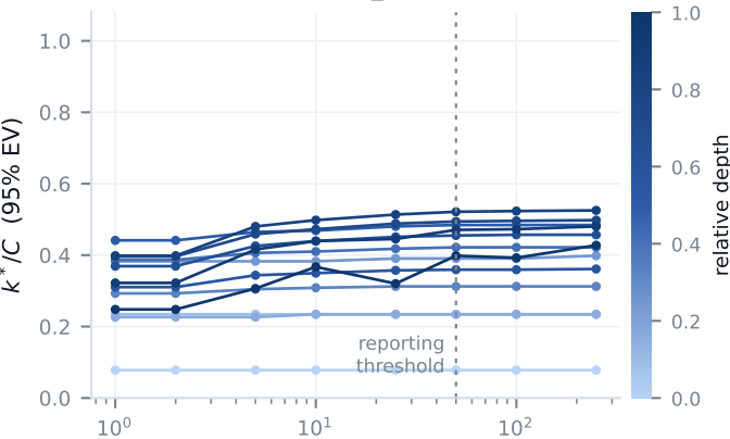
vgg16_bn
