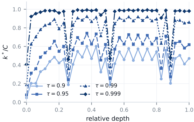
timm_resnet34.a1_in1k
