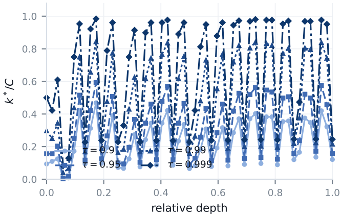
timm_resnet50.gluon_in1k
