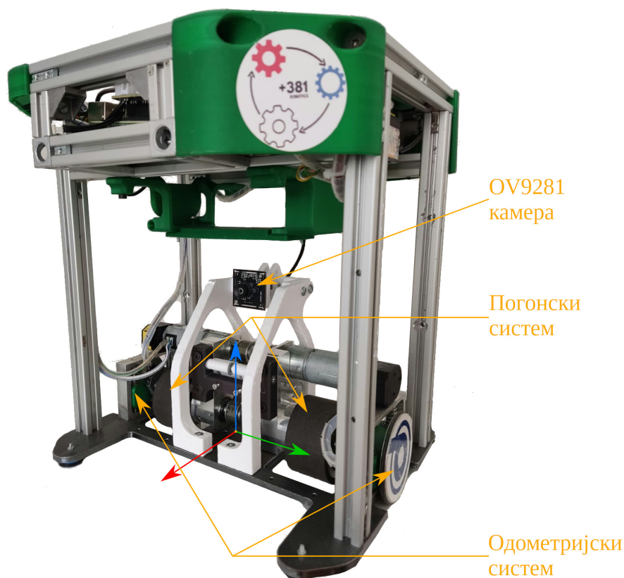
Слика 3.1 Робот тима +381 Robotics који је коришћен за прикупљање скупа података
