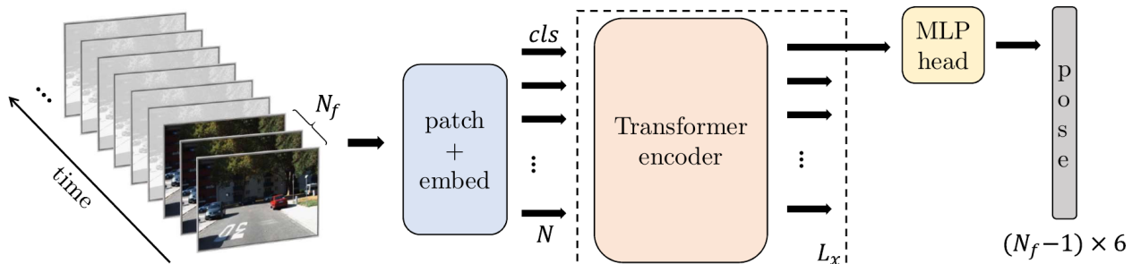
Слика 2.4 Структура модела TSformer-VO (преузето из [17])
