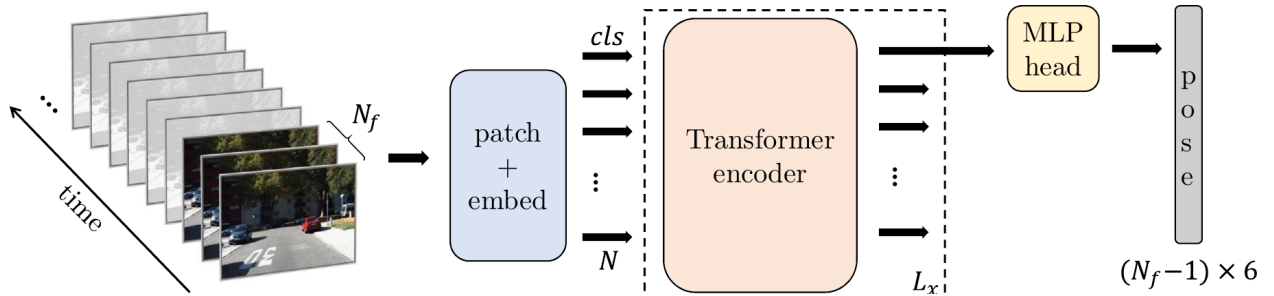
Слика 2.4 Структура модела TSformer-VO (преузето из [17])
