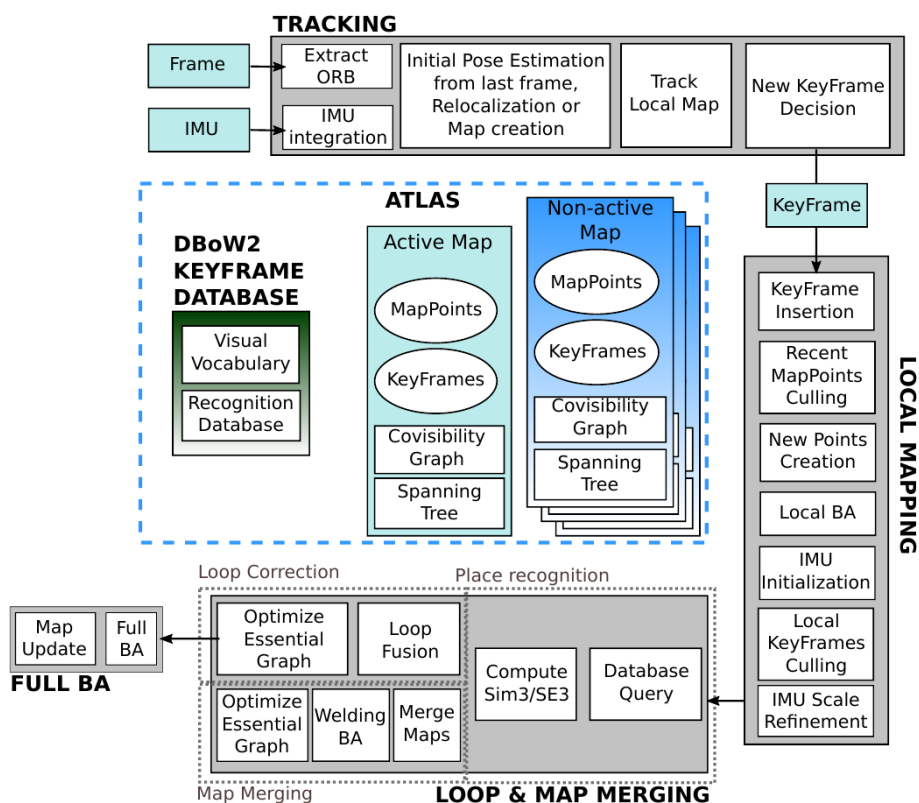
Слика 2.3 Компоненте система ORB-SLAM3 (преузето из [14])
