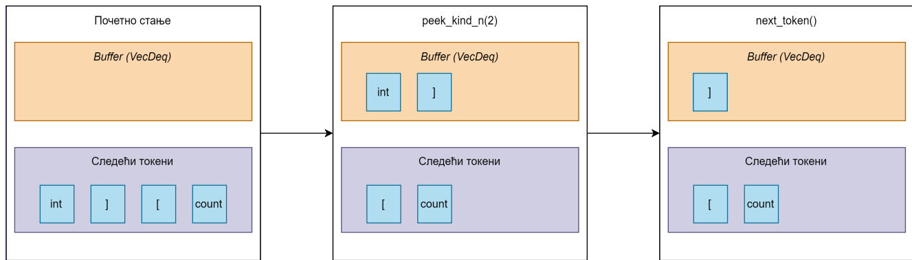
Слика 13: Управљање интерним бафером током вирења унапред.
