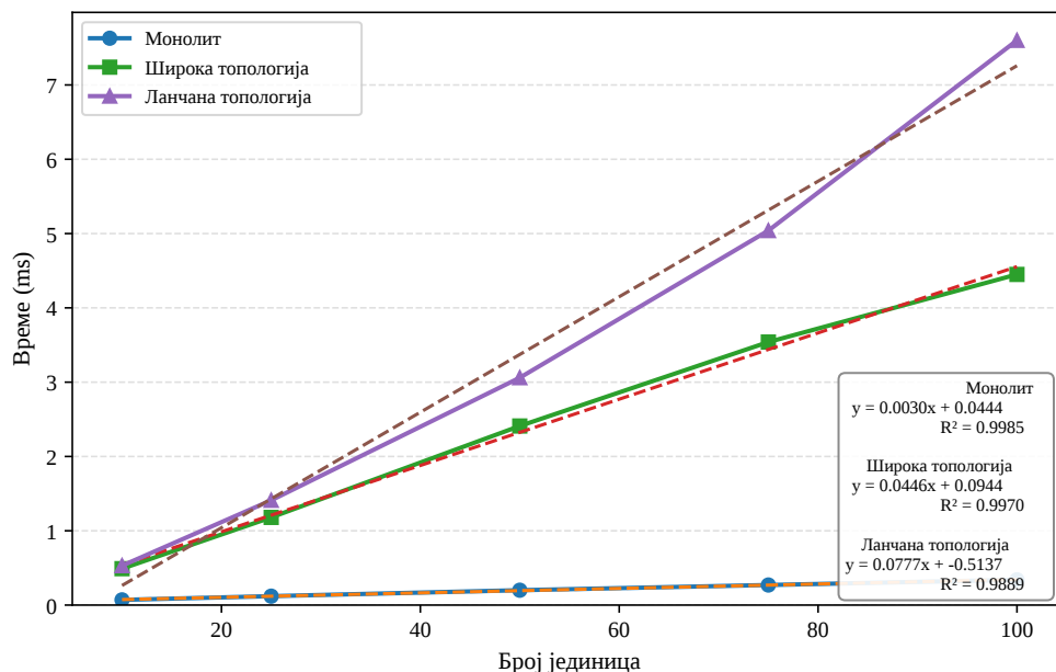
Слика 16: Линеарна зависност времена превођења од броја модула за различите топологије.
