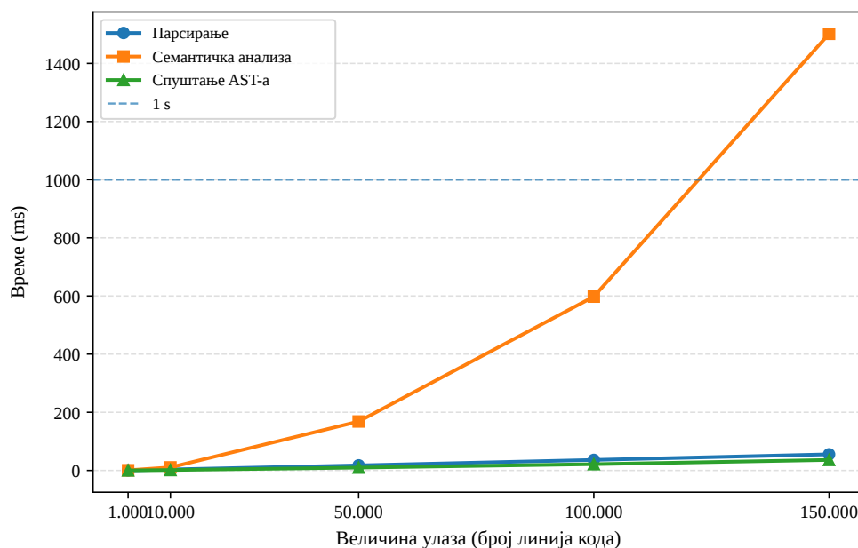
Слика 15: Зависност времена извршавања фаза превожјења од броја линија кода
