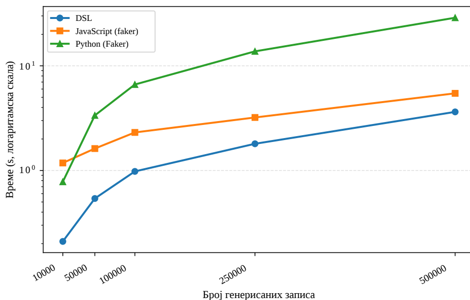
Слика 18: Зависност времена генерисања од броја записа.
