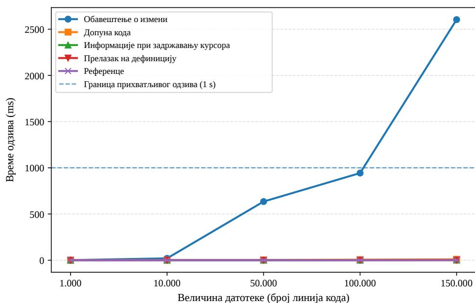
Слика 19: Зависност времена одзива LSP операција од величине датотеке.
