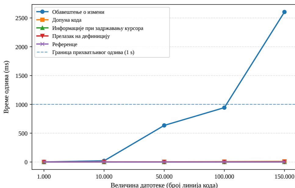
Слика 14: Зависност времена одзива LSP операција од величине датотеке.
