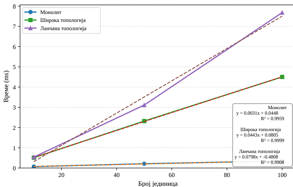
Слика 13: Линеарни тренд времена превођења у функцији броја модула.
