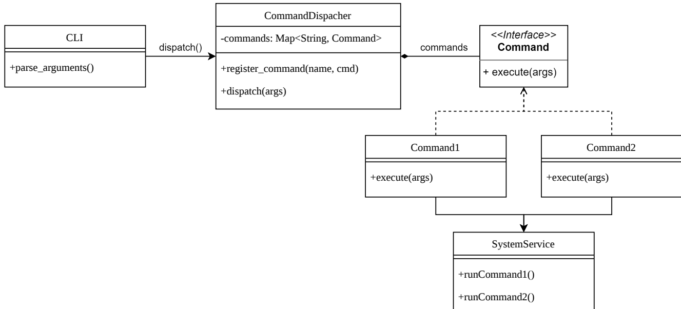
Слика 7: Структура дизајнерског шаблона диспечер команди.
