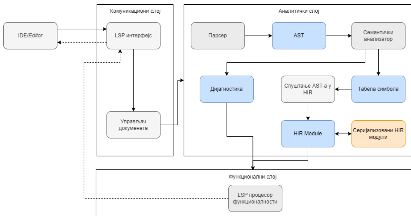
Слика 7: Архитектура LSP система и ток обраде LSP захтева.
