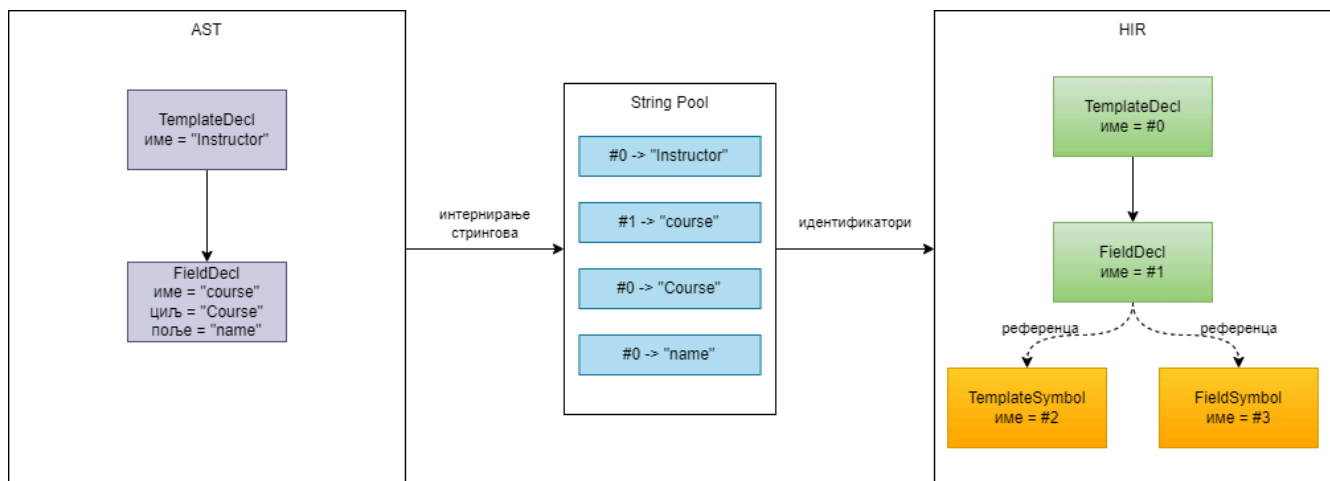
Слика 2: Поређење AST-а и HIR-а на примеру декларације шаблона.
