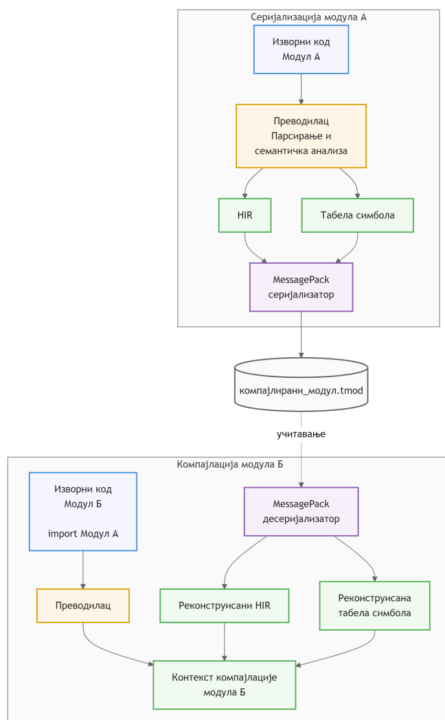
Слика 3: Процес серијализације компајлираног модула и његовог увоза током компајлације.
