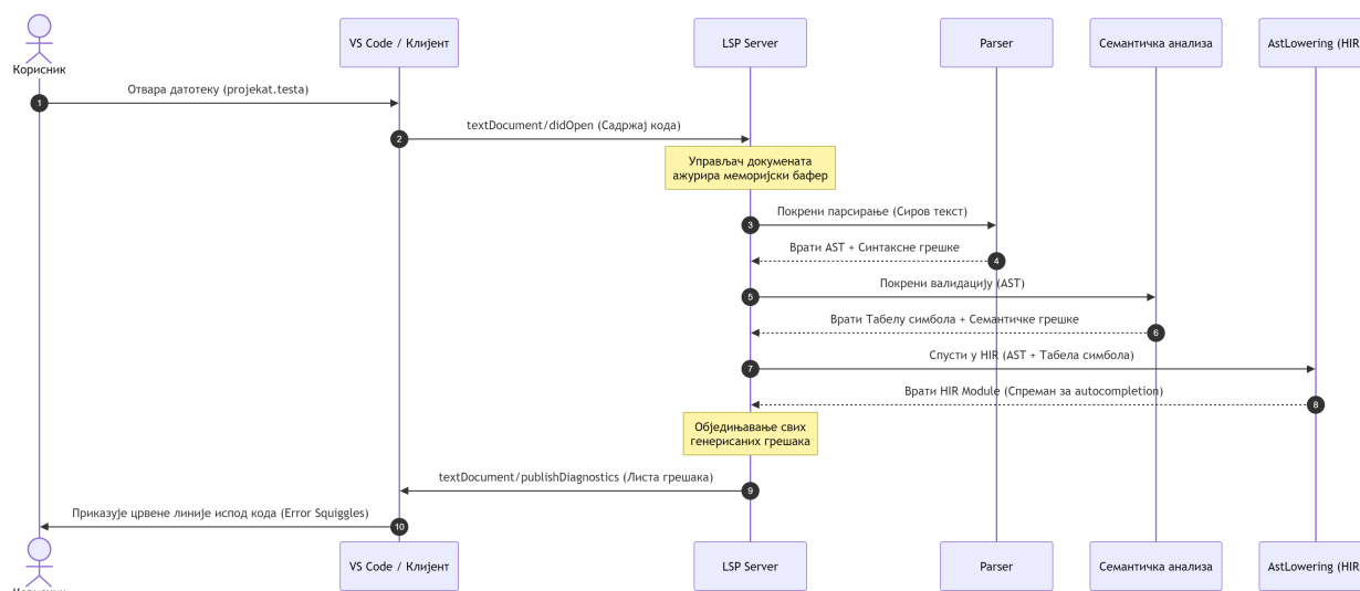
Слика 8: Секвенцијални дијаграм обраде догађаја при отварању датотеке
