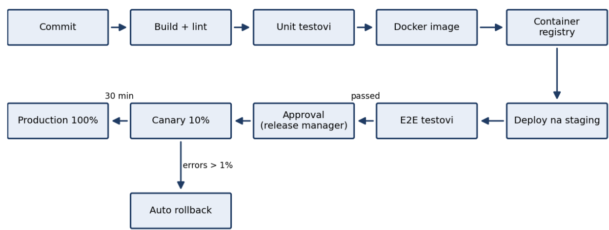
Slika 1. Faze pipeline-a
