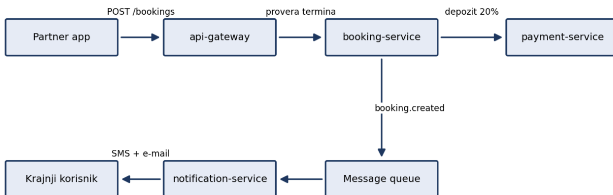
Slika 1. Tok nove rezervacije
