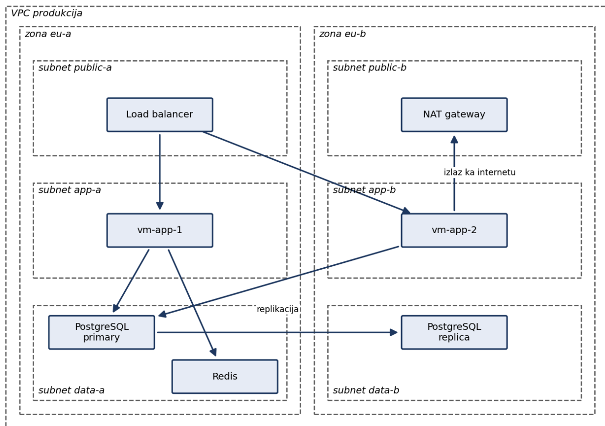
Slika 1. Raspored komponenti produkcije
