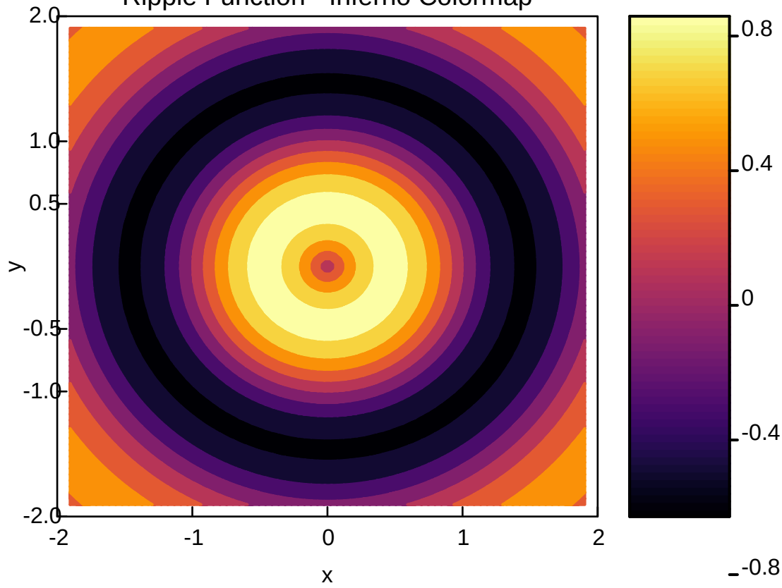
Ripple Function - Inferno Colormap
