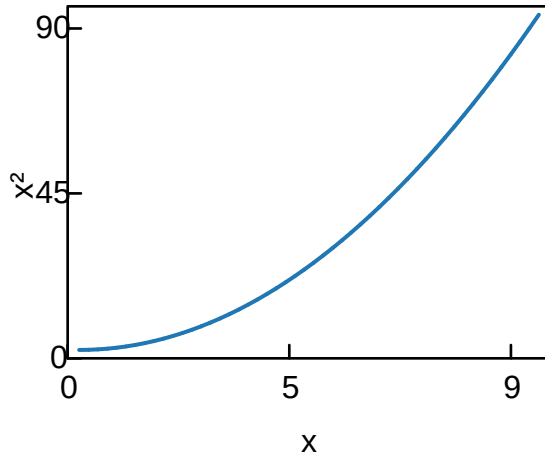
Quadratic
