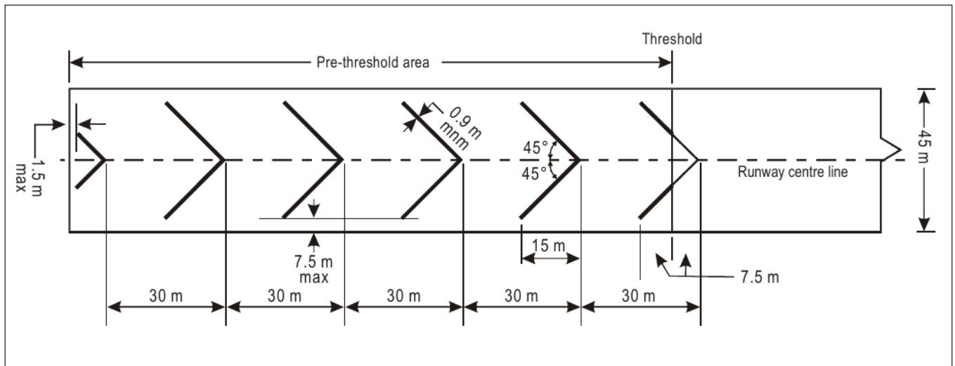
ICAO Annex14, 图7-3, 印刷页7-7, PDF第245页: 前入口不可正常使用铺筑区域的V形图示。[A14]
