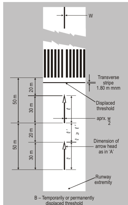
ICAO Annex14, 图5-4(B), 印刷页5-9, PDF第135页: 内移入口横条与白箭头。[A14]
