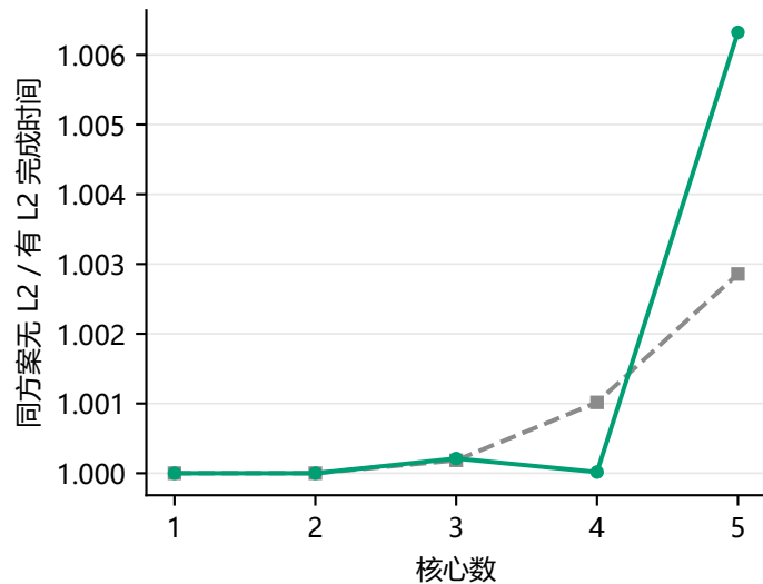
(c) 场景 B + 只读 Cache
