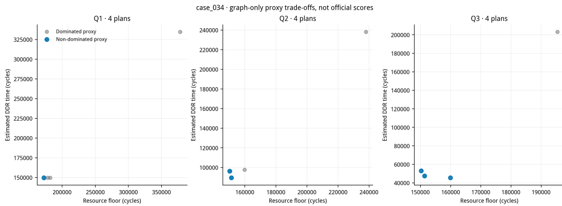
图 5-7 图结构候选的代理目标 Pareto 对比
