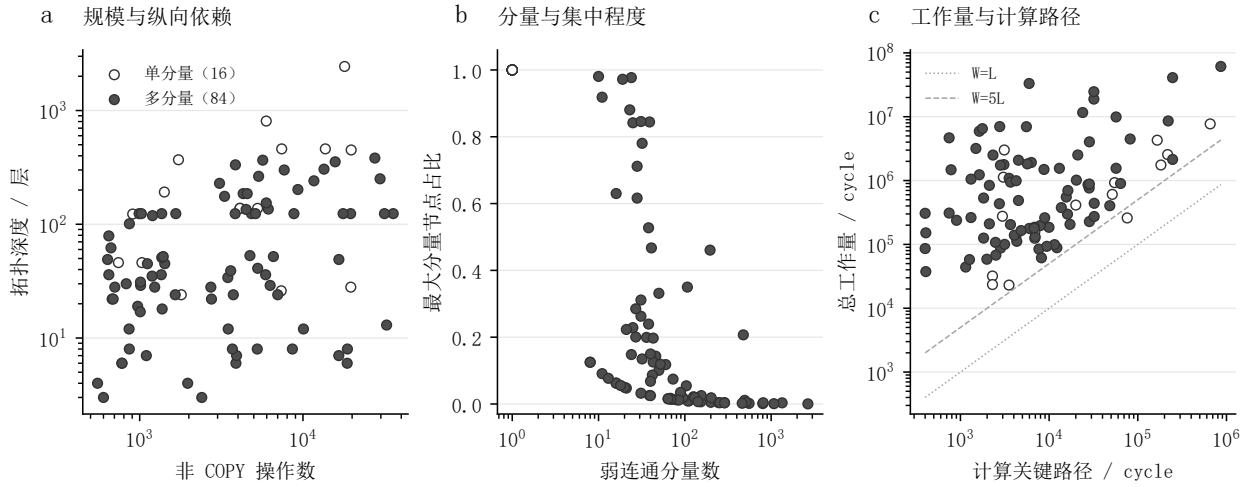
图 5-1 100 图的结构与工作量差异，每个点代表一张原始图。a 操作规模与拓扑深度；b 分量数与最大分量节点占比；c 计算关键路径与总工作量，参考线表示 W = L 和 W = 5L 。空心、实心符号区分单分量和多分量图。对数坐标用于展示数量级跨度，不改变特征计算。
