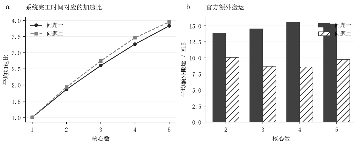
图 7-2 两种场景的全量结果比较。左图为逐图加速比的算术平均，单核值按定义为 1；右图为官方统计的平均新增 DDR 字节数，以 MiB 表示。除单核定义值外，每个点或柱均对应 100 个计算图。
