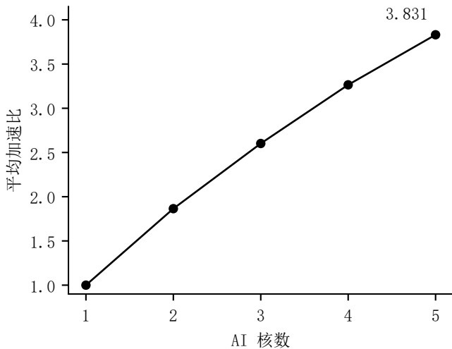
(a) 核数与平均加速比
