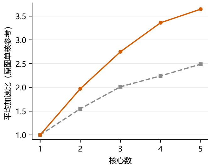
(b) 场景 B: 同核复用
