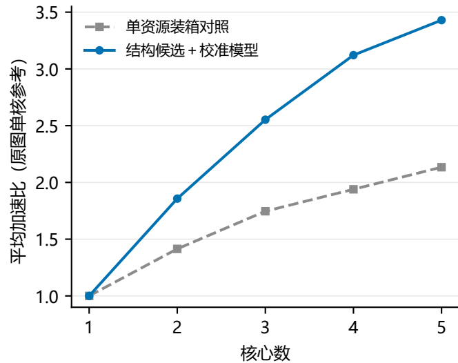
(a) 场景 A: Task 边界
