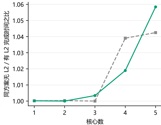
(c) 场景 B + 只读 Cache
