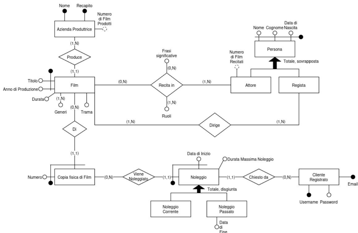
Figura 1: Schema Entità-Relazioni
